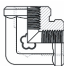
A07 雙內牙彎頭 Union Elbow
