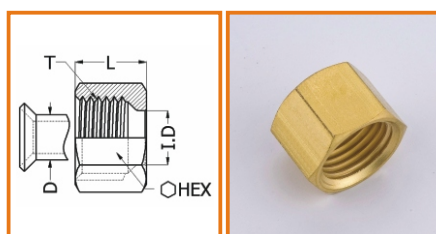
平口螺帽 Short Nut
