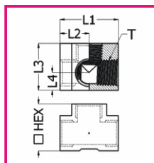
立型四通 Stand-type Cross
