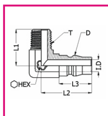
快速彎頭 Quick Coupling Elbow
