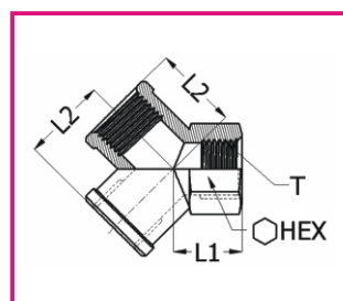
內牙 Y 型三通 Y type Union Tee
