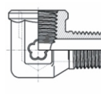
A06 內外牙彎頭 Street Elbow
