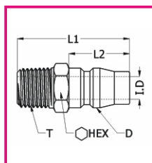
快速接頭 Quick Coupling Connector
