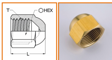
螺帽蓋 Cap Nut
